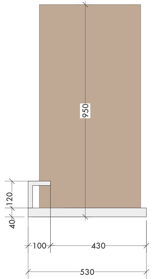
Sezione_scala 1:10
